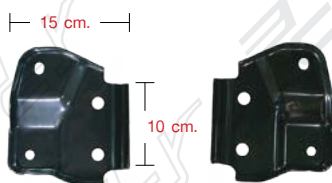
BUMPER STAY LH/RH (N) ขากันชน ซ้าย/ขวา (หัวแคบ)
